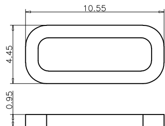
防水圈图
